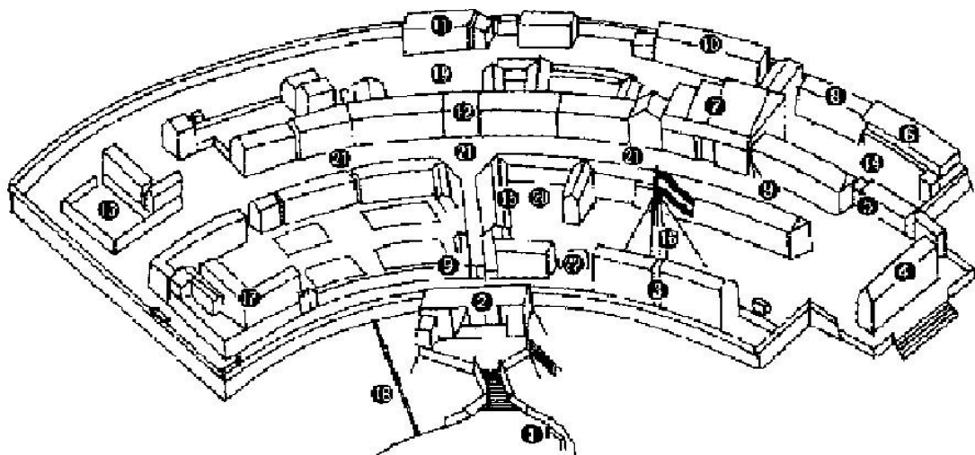
图 1 出岛结构图
